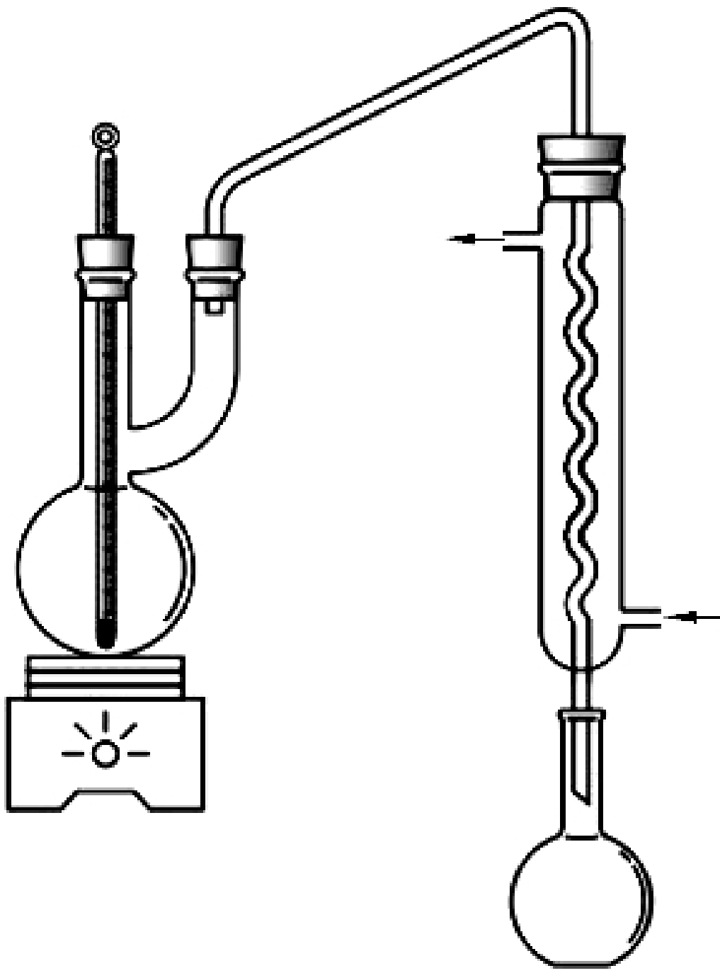
图 3 氟化物蒸馏装置
