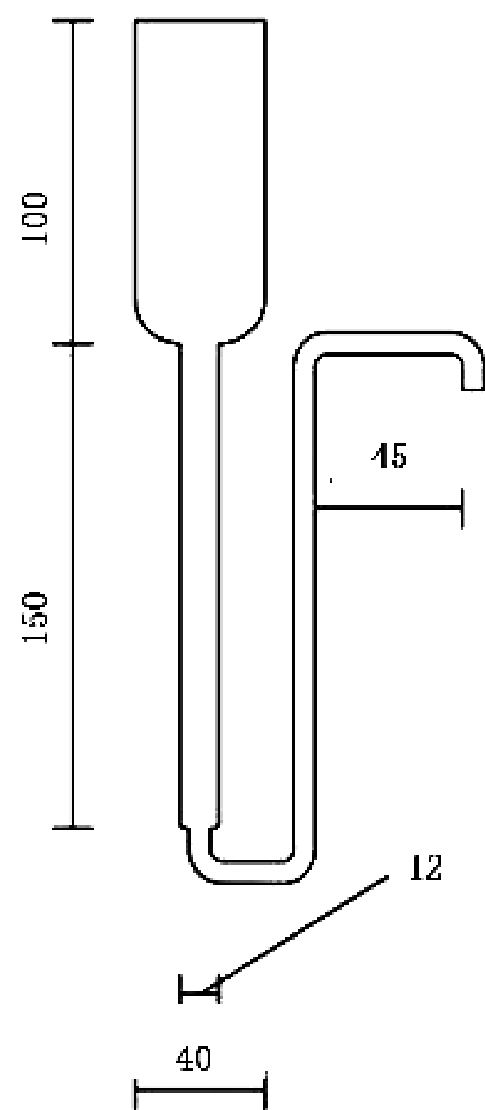
图 2 离子交换柱
