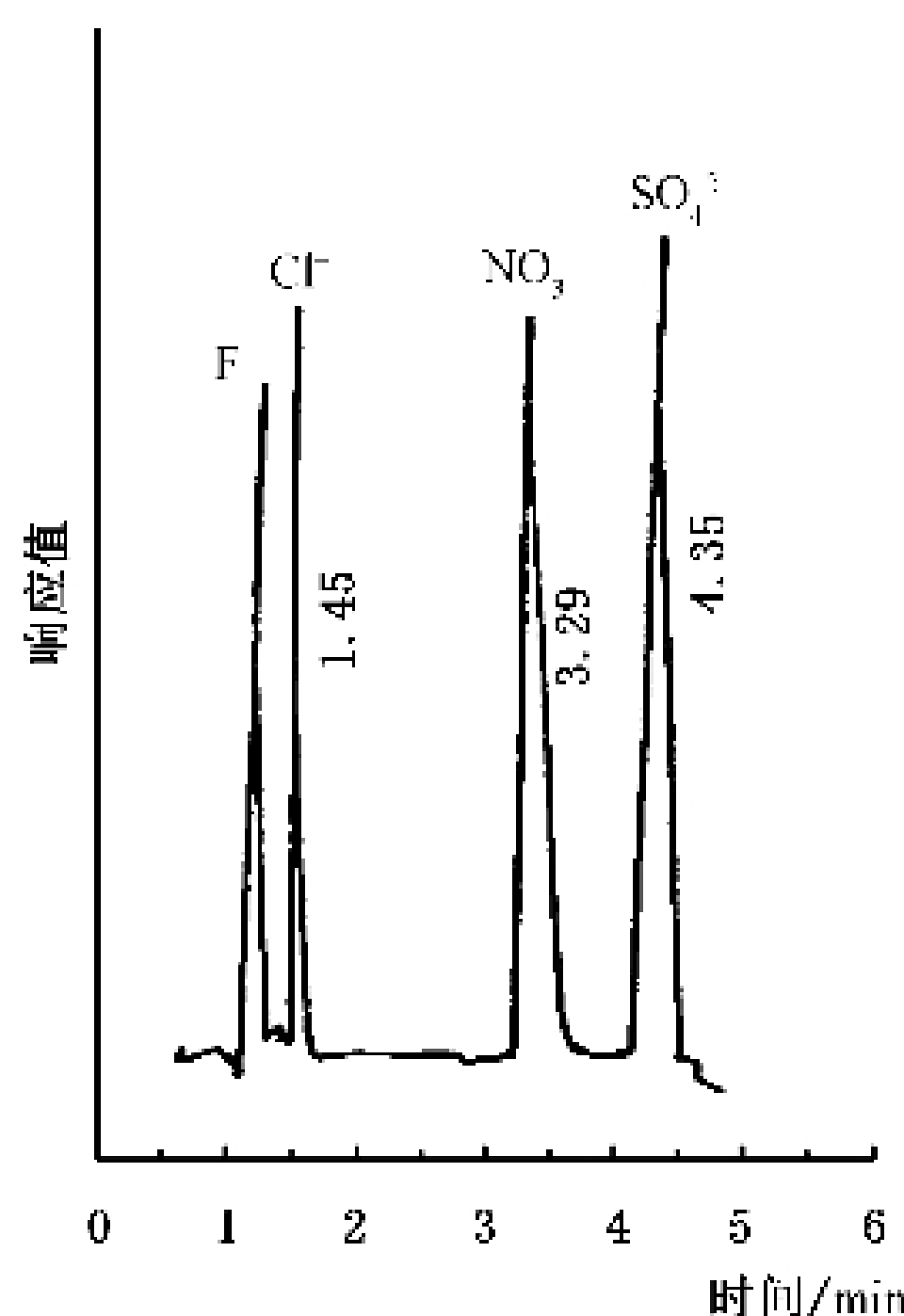
图 1 离子色谱图
